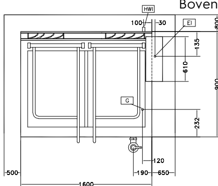
Boven aanzicht
